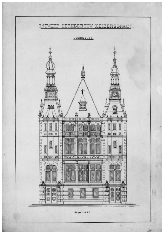
Ontwerptekening Keizersgrachtkerk (Tjeerd Kuipers)
